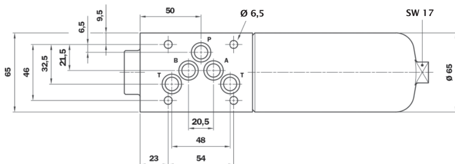
G1: CETOP-Lochbild, NG 10, Filtertopf rechts
